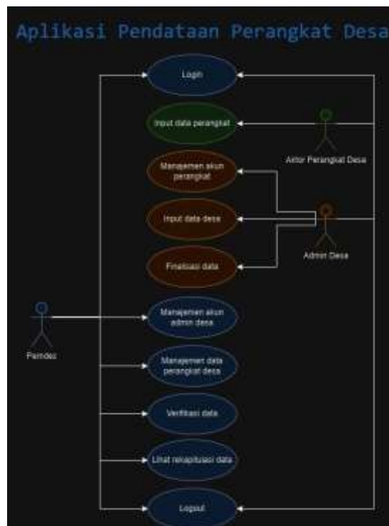
Gambar 5 Usecase pada Website Perangkat Desa
